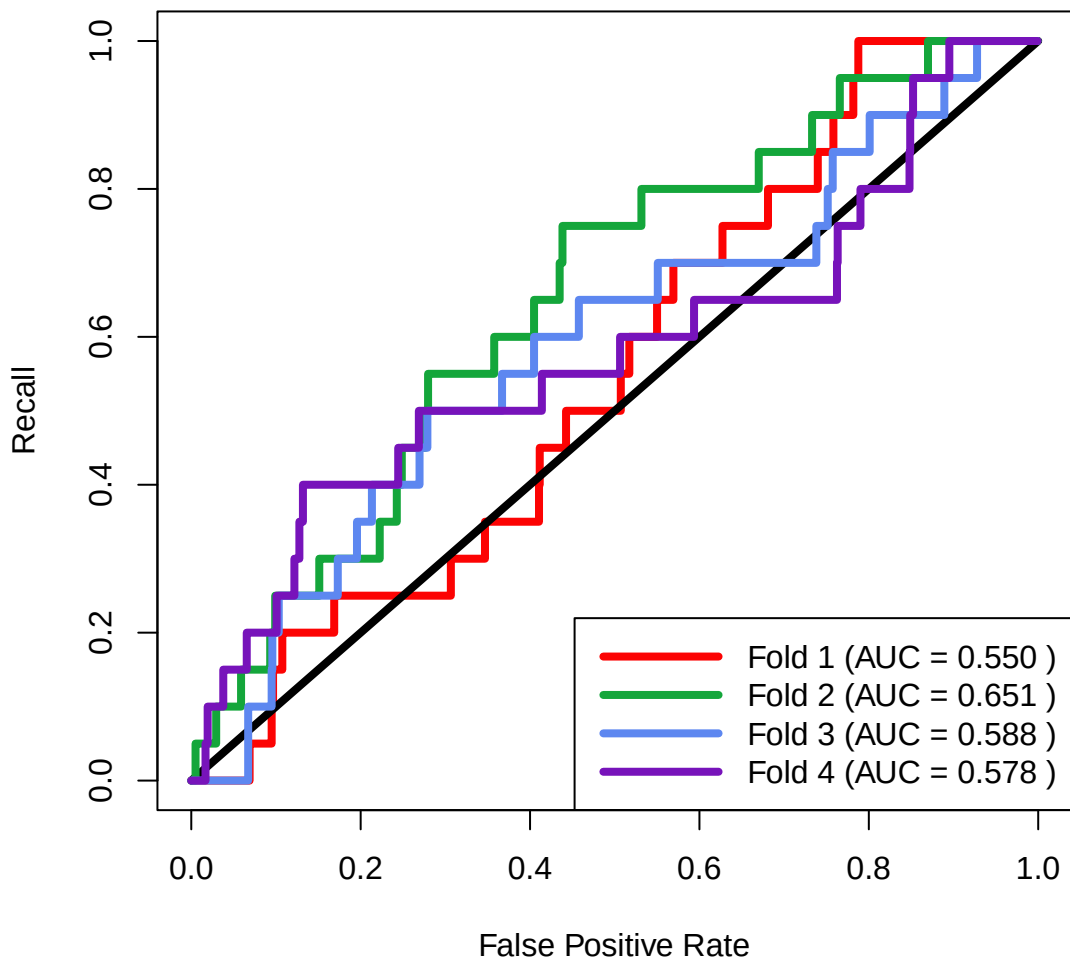
Primig 2000 Dataset 2: 24x20x8x1 Validation
